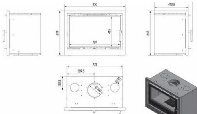
Fig. 5. ARKE cassette – dimensiones
