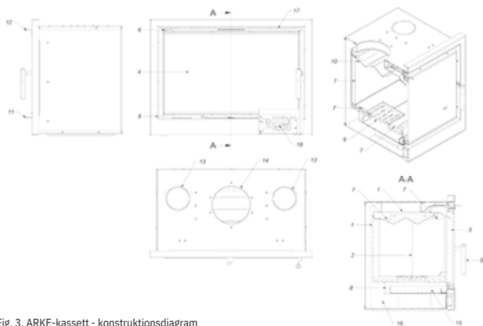
Fig. 3. ARKE-kassett - konstruktionsdiagram
